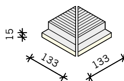
YTTERHÖRN C YTA 133x133x40 mm
