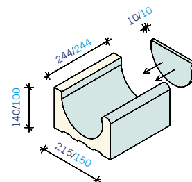
BRED SKVALPRÄNNA MED AVSLUT HÖGER 215x244x140 mm
