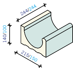
BRED SKVALPRÄNNA 215x244x140 mm
