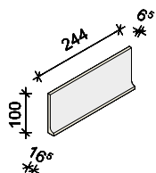
SOCKEL SLÄT R10/B 244x100x6,5 mm
