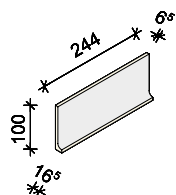
SOCKEL 244x100x6,5 mm 66 4000 690 Oglaserad 66 4000 901 Vit matt 66 4000 900 Vit blank 66 4000 + FC
