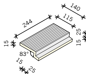
UPPLAGSPLATTA C YTA 140x244x40 mm
