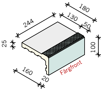
GREPPKANTSPLOTTA C YTA 180x244x100 mm
