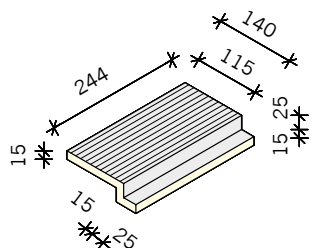
UPPLAGSPLATTA C YTA 140x244x40 mm
