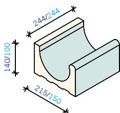
BRED SKVALPRÄNNA INNERHÖRN 215x208x140 mm
