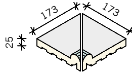
INNERHÖRN C YTA 173x173 mm
