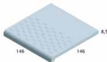
TRAPPNOS 146x146x8 mm Artikel ST 15
