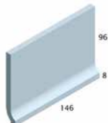
HÅLKÄL 96x146x8 mm Artikel SB 15
