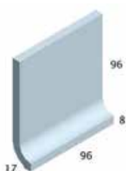
HÅLKÄL 96x96x8 mm Artikel SB
