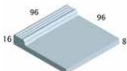
GREPPKANTSPLATTA 96x96x8 mm Artikel PES
