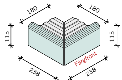
YTTERHÖRN 180x238x115 mm
