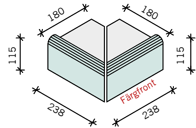
YTTERHÖRN C YTA 180x238x115 mm
