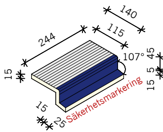
UPPLAGSPLATTA C YTA 140x244x65 mm
