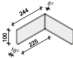
INNERHÖRN 244x100x6,5 mm 66 4002 690 Oglaserad 66 4002 901 Vit matt 66 4002 900 Vit blank 66 4000 + FC
