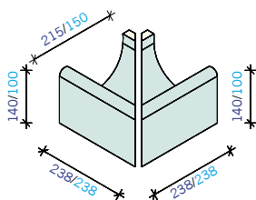
BRED SKVALPRÄNNA YTTERHÖRN 215x238x140 mm
