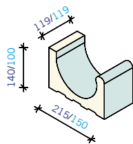
BRED SKVALPRÄNNA KORT 215x119x140 mm
