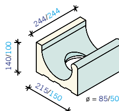
BRED SKVALPRÄNNA MED UTLOPP 215x244x140 mm
