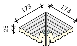
INNERHÖRN 173x173 mm
