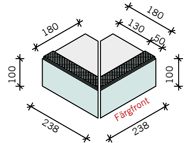
YTTERHÖRN C YTA 180x238x100 mm
