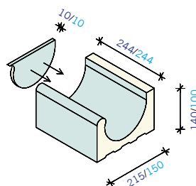
BRED SKVALPRÄNNA MED AVSLUT VÄNSTER 215x244x140 mm
