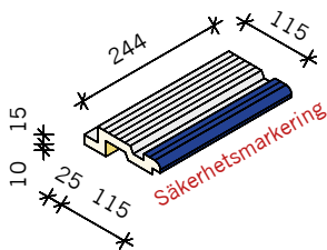
GREPPKANTSPLATTA C YTA 115x244 mm
