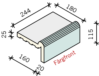
GREPPKANTSPLOTTA C YTA 180x244x115 mm
