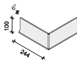
YTTERHÖRN 244x100x6,5 mm
