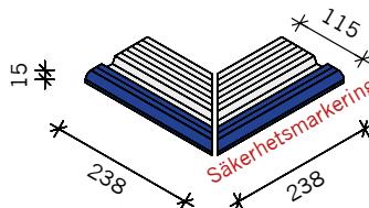
YTTERHÖRN C YTA 115x238 mm
