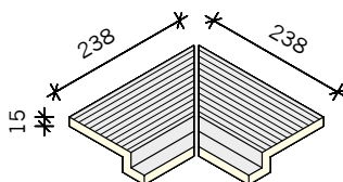
INNERHÖRN C YTA 238x238x40 mm
