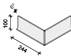
YTTERHÖRN 244x100x6,5 mm 66 4007 690 Oglaserad 66 4007 901 Vit matt 66 4007 900 Vit blank 66 4000 + FC
