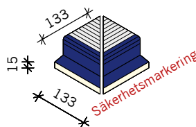
YTTERHÖRN C YTA 133x133x65 mm
