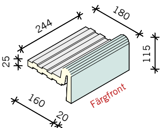
GREPPKANTSPLOTTA 180x244x115 mm
