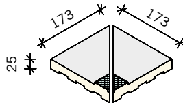
INNERHÖRN C YTA 173x173 mm
