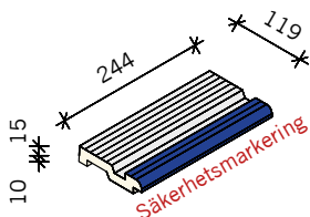
GREPPKANTSPLATTA C YTA 119x244 mm
